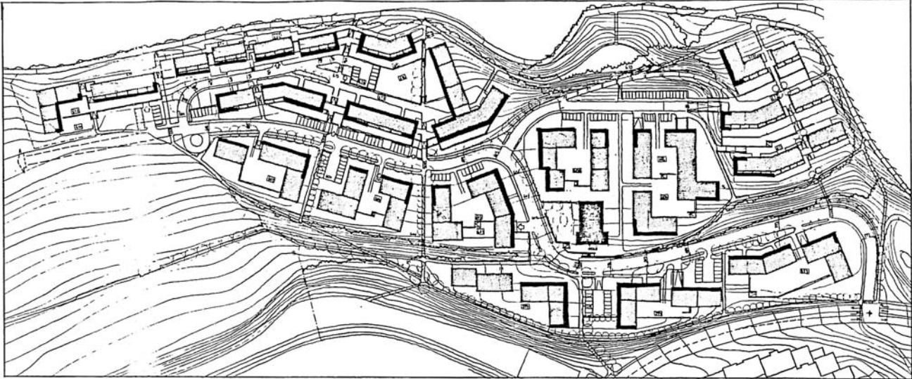
Abb. 24: Weitere Modifikationen der Konzeptvariante 2
